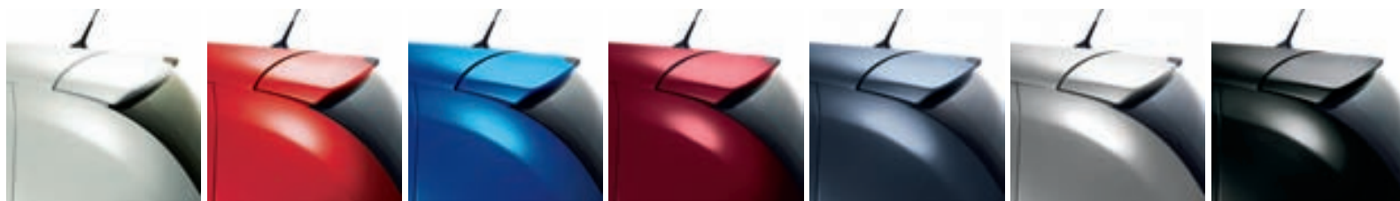
BLANC GLACIER (OV 369)
